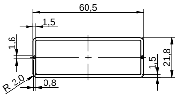
0,5 Recommended Tin Paste Mask Layer
