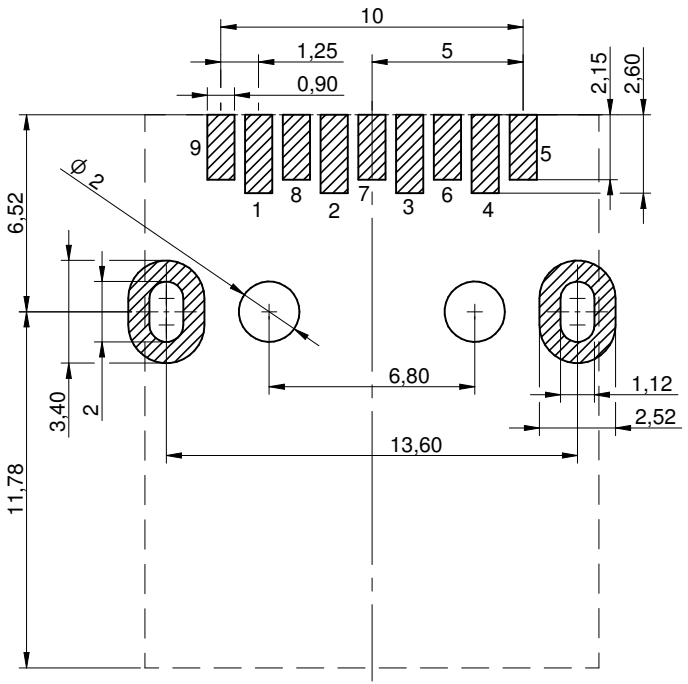
General tolerance ±0,05
