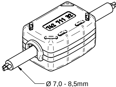
Scale - 1:1,25
