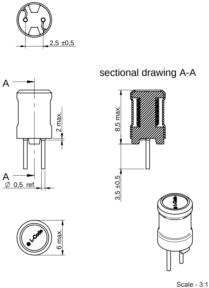
Scale - 3:1
